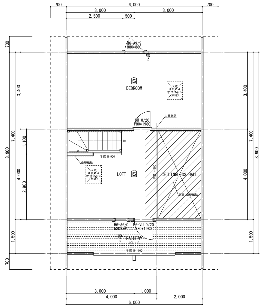
2 階平面図 S=1/50 ※雨樋・網戸オプション
