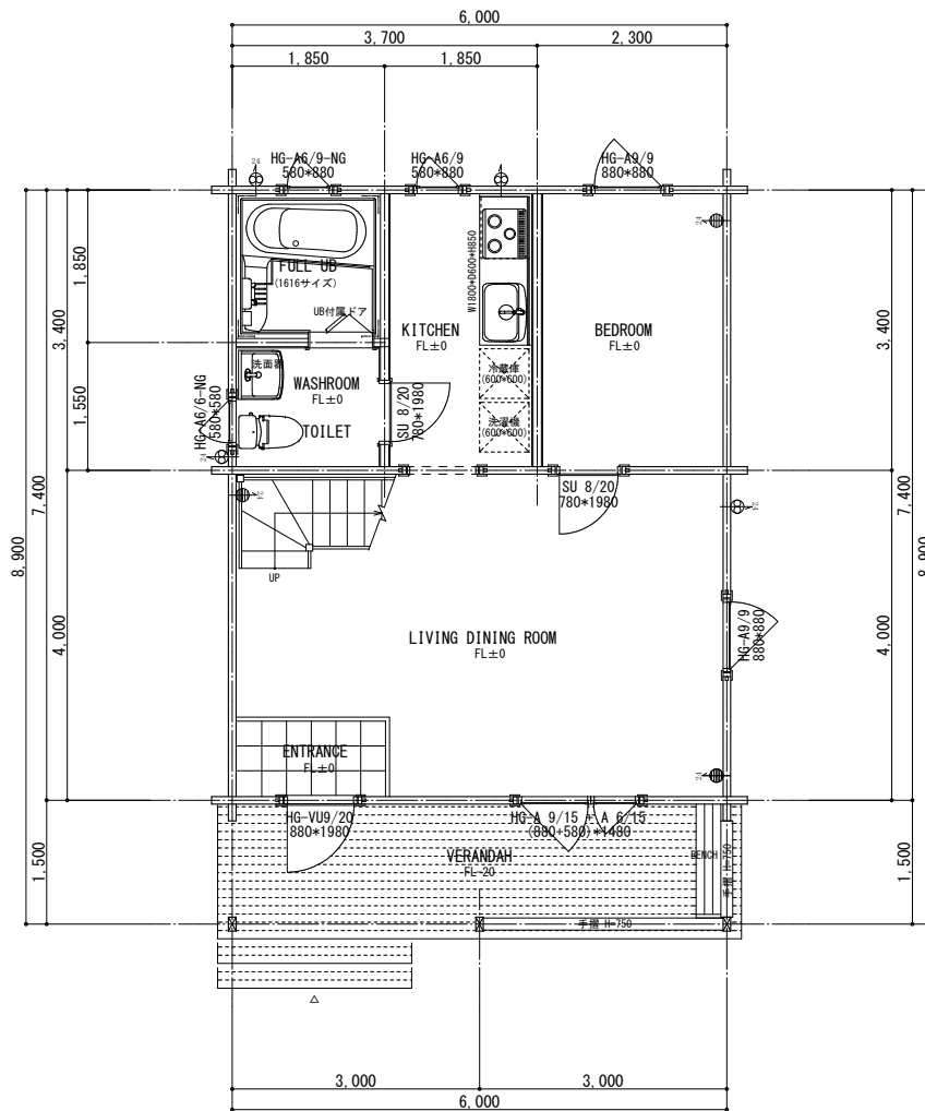
1 階平面図 S=1/50 ※雨樋・網戸オプション
